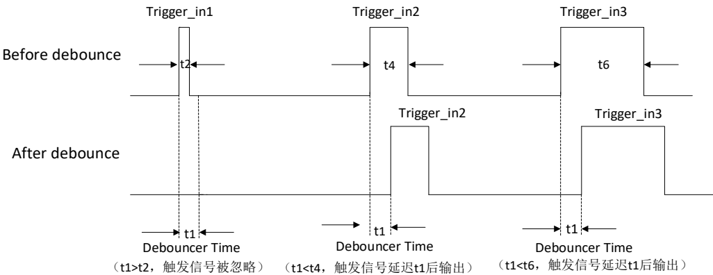
图3-45 触发输入信号去抖时序
