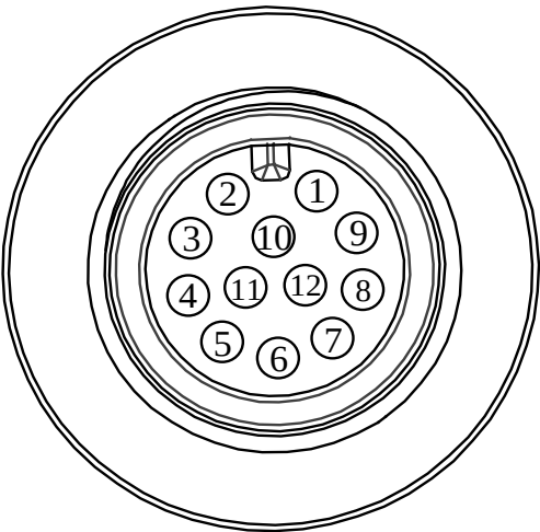
图1-5 12-pin 接口
