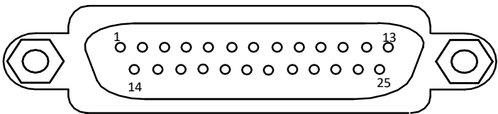
图4-12 25-pin 公头连接器
