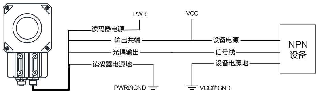
图4-9 输出信号接 NPN 设备（不使用上拉电阻）
