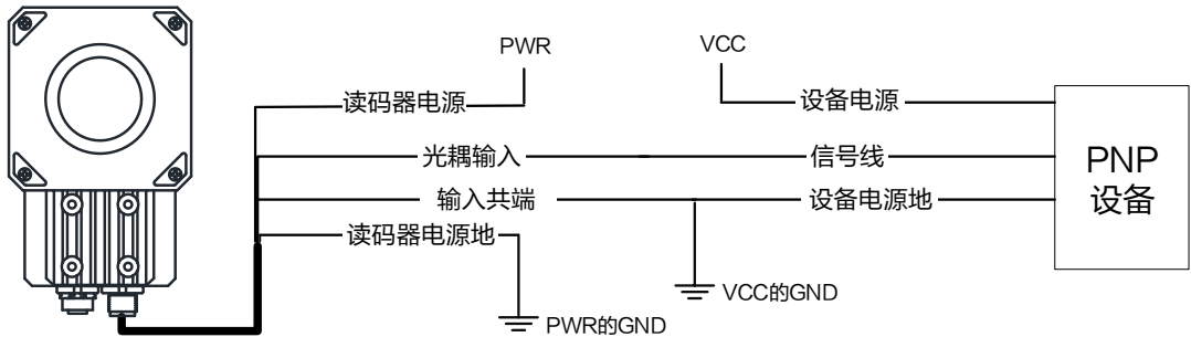
图4-5 输入信号接 PNP 设备
