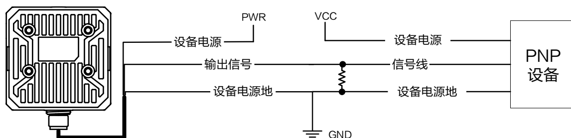
图5-8 输出信号接 PNP 设备
