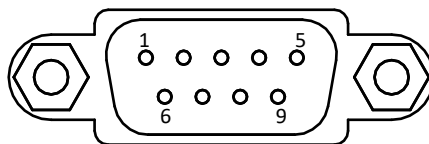
图5-10 9-pin 公头连接器
