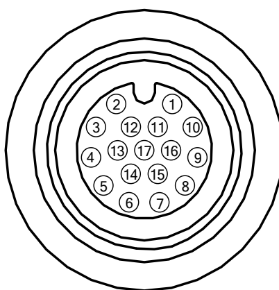
图2-3 17-pin M12 接口
