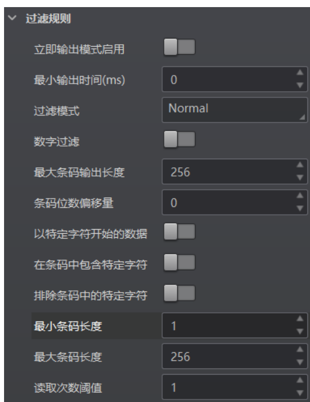
图4-81 普通过滤模式过滤规则参数
