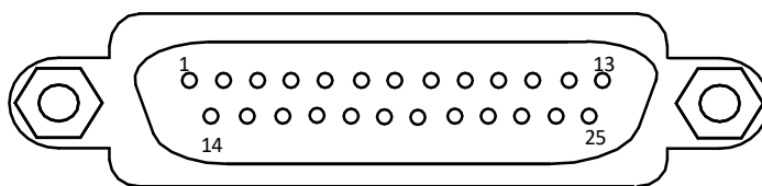
图5-12 25-pin 公头连接器
