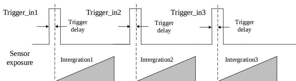
图4-41 信号延迟原理
