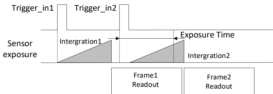
图4-44 第2帧曝光移动处理时序
