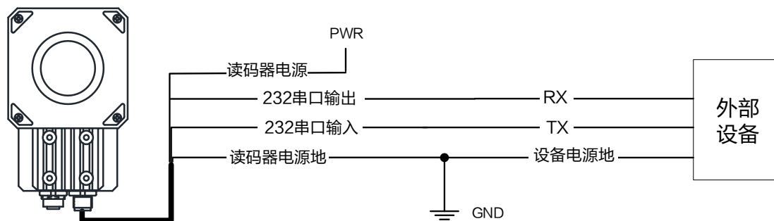
图5-13 RS-232 串口接线
