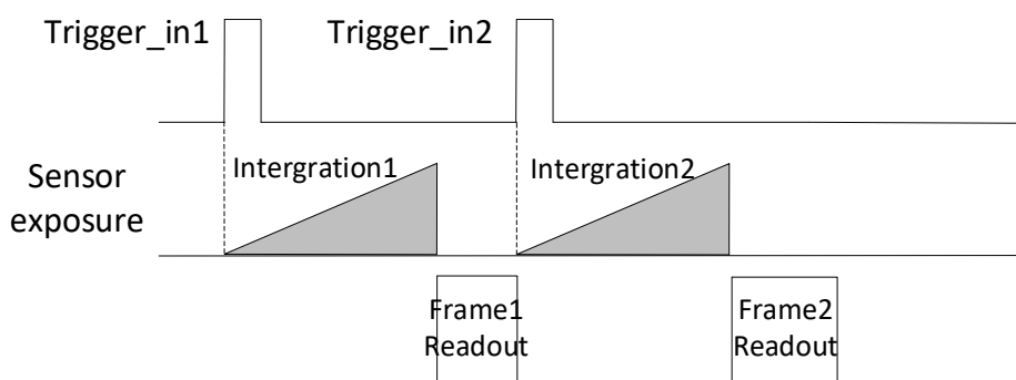
图4-42 第1帧被强制结束时序
