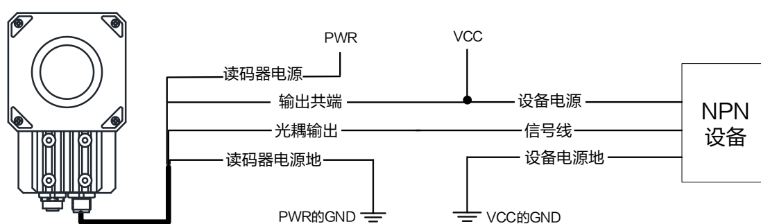
图5-9 输出信号接 NPN 设备（不使用上拉电阻）
