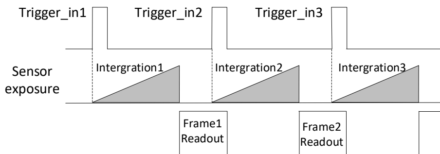
图4-43 第2帧正常处理时序
