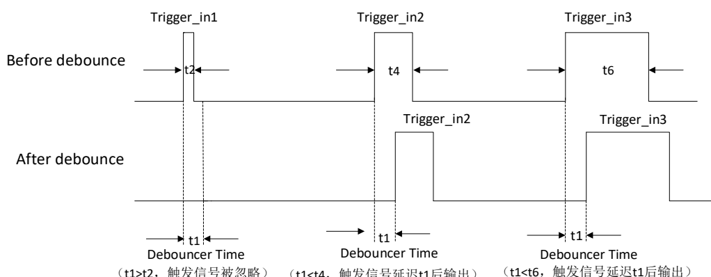
图4-47 触发输入信号去抖时序
