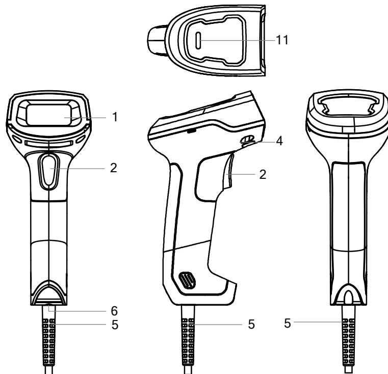
图2-4 四系列设备外观
