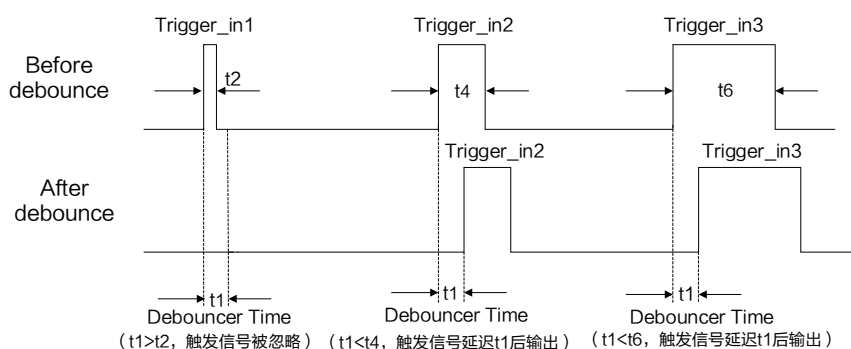
图4-20 触发输入信号去抖时序
